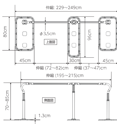
ロング2050伸縮タイプ 片手すり XPN-L80615
