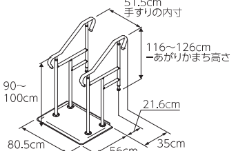
2-2 あがりかまち高さ20~40cm対応
